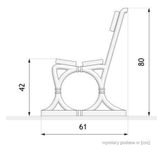
wymiar podane w [cm]
