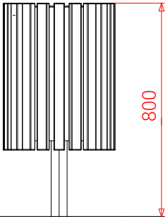
WIDOK Z FRONTU
