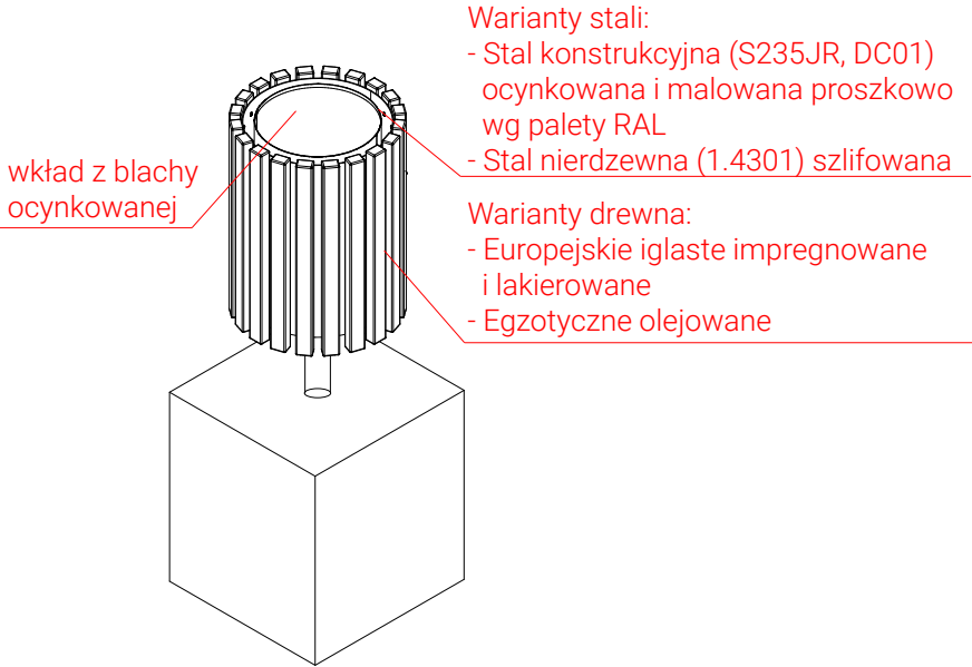
RZUT IZOMETRYCZNY
