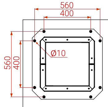
ESPACEMENT DES TROUS DE MONTAGE (FRAIS GÉNÉRAUX)
