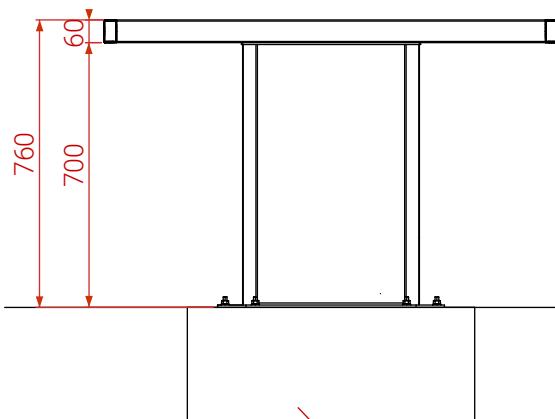
VUE FRONTALE
