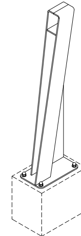
RZUT IZOMETRYCZNY
