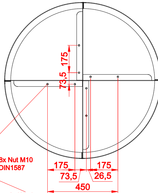
ESPACEMENT DES TROUS DE MONTAGE
