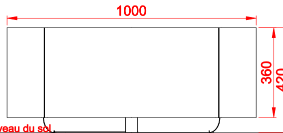
VUE LATÉRALE
