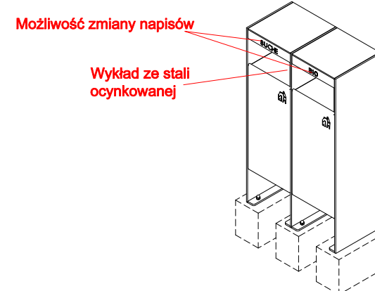
RZUT IZOMETRYCZNY
