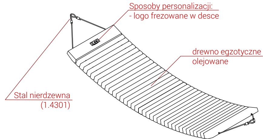
RZUT IZOMETRYCZNY
