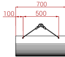
WIDOK Z FRONTU
