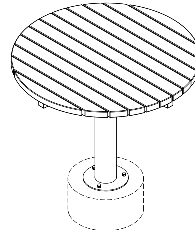
RZUT IZOMETRYCZNY
