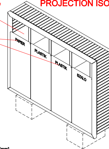
PROJECTION ISOMÉTRIQUE
