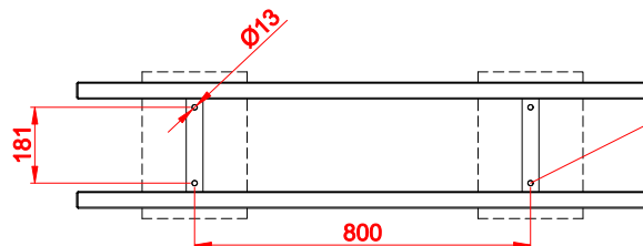
ESPACEMENT DES TROUS DE MONTAGE
