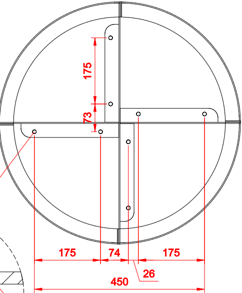
ROZSTAW OTWORÓW MONTAŻOWYCH
