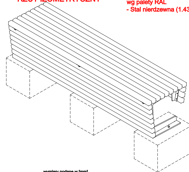
RZUT IZOMETRYCZNY
