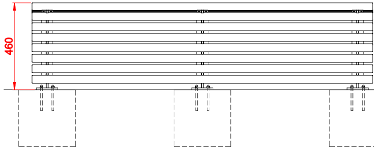
WIDOK Z FRONTU
