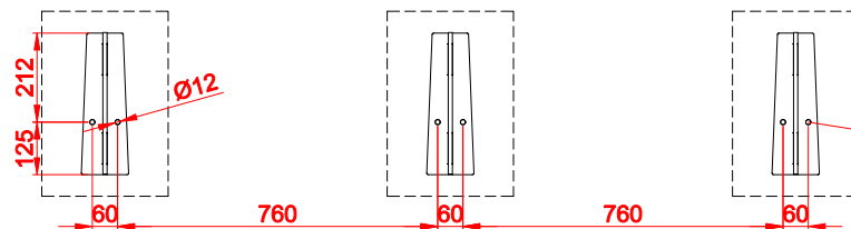
ROZSTAW OTWORÓW MONTAŻOWYCH
