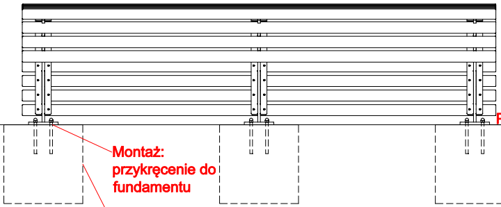
WIDOK Z TYŁU
