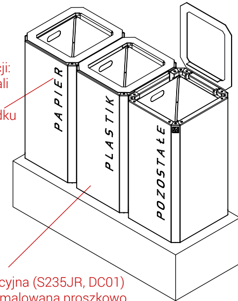
RZUT IZOMETRYCZNY
