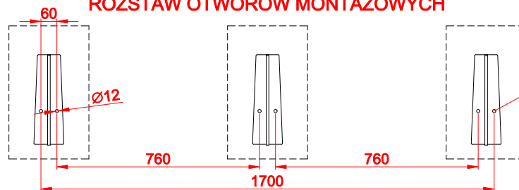
ROZSTAW OTWORÓW MONTAŻOWYCH
