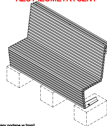
RZUT IZOMETRYCZNY
