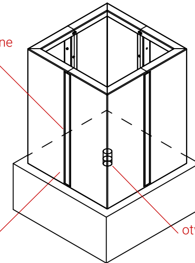
RZUT IZOMETRYCZNY
