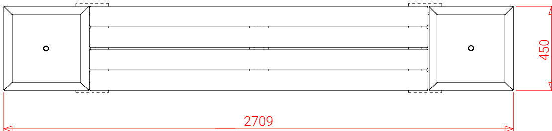
WIDOK Z GÓRY
