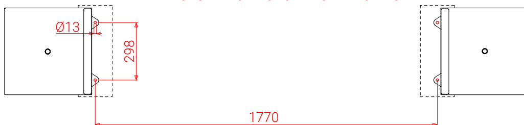
ROZSTAW OTWORÓW MONTAŻOWYCH
