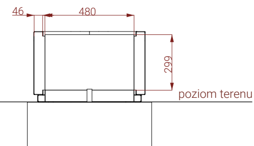
PRZĘKRÓJ
