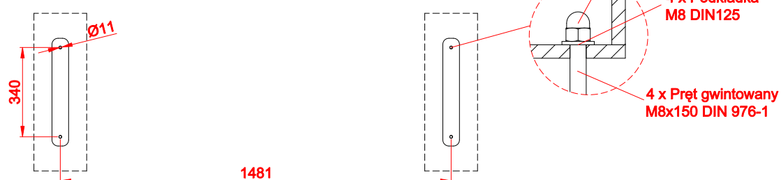
ROZSTAW OTWORÓW MONTAŻOWYCH
