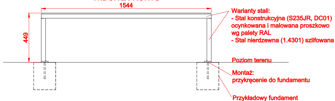
WIDOK Z FRONTU
