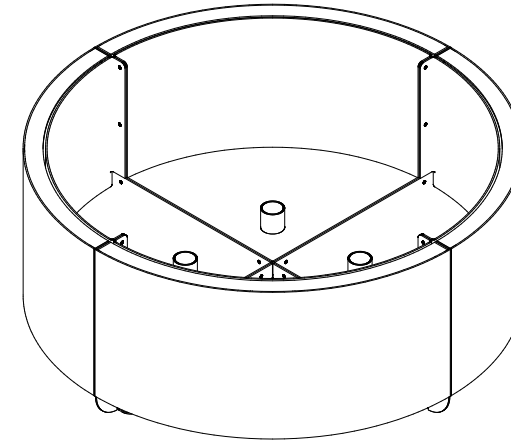
RZUT IZOMETRYCZNY
