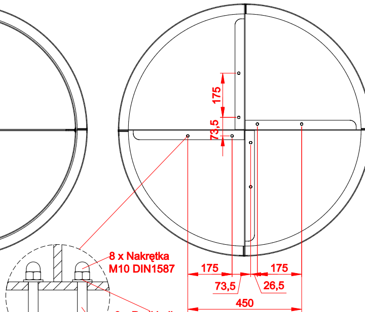
ROZSTAW OTWORÓW MONTAŻOWYCH
