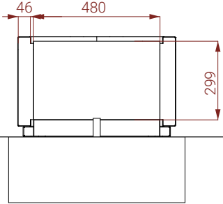
PRZEKRÓJ
