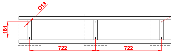
ROZSTAW OTWORÓW MONTAŻOWYCH
