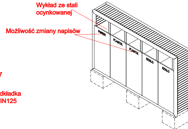
RZUT IZOMETRYCZNY
