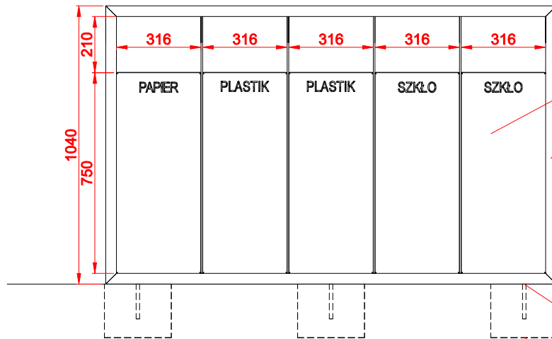
WIDOK Z FRONTU
