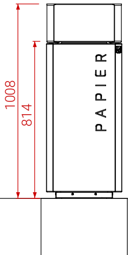
VUE FRONTALE
