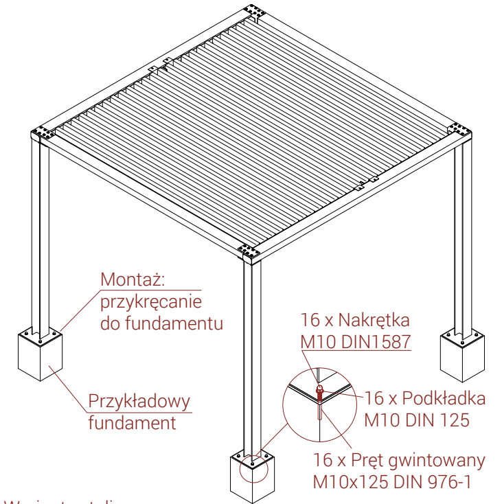
RZUT IZOMETRYCZNY
