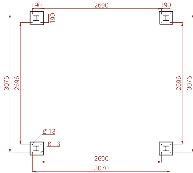
ROZSTAW OTWORÓW MONTAŻOWYCH
