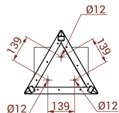
ROZSTAW OTWORÓW MONTAŻOWYCH
