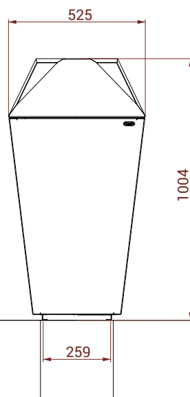
WIDOK Z PRZODU
