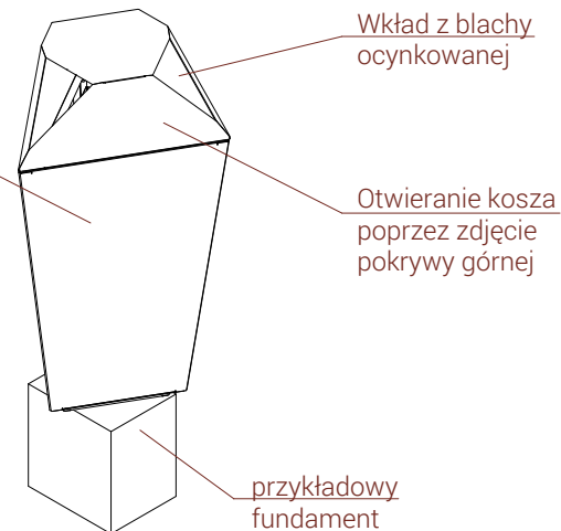
RZUT IZOMETRYCZNY
