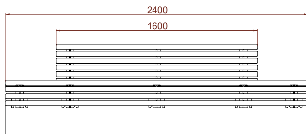
WIDOK Z PRZODU
