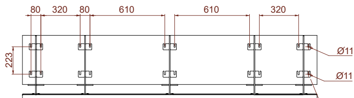
ROZSTAW OTWORÓW MONTAŻOWYCH WIDOK Z GÓRY
