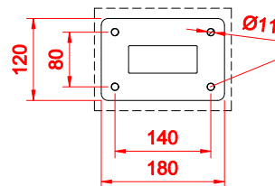
ROZSTAW OTWORÓW MONTAŻOWYCH
