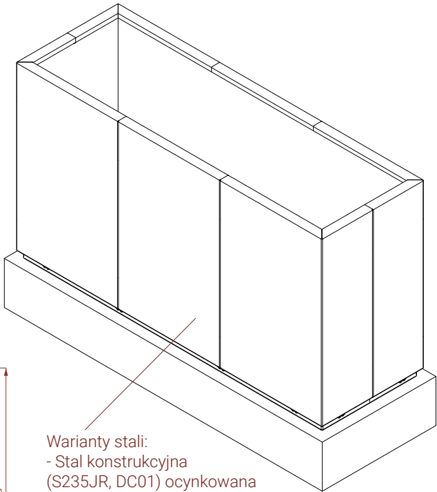
RZUT IZOMETRYCZNY
