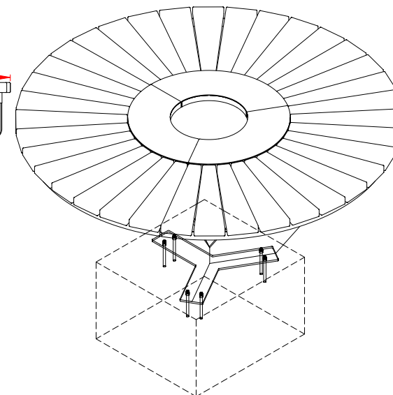
RZUT IZOMETRYCZNY
