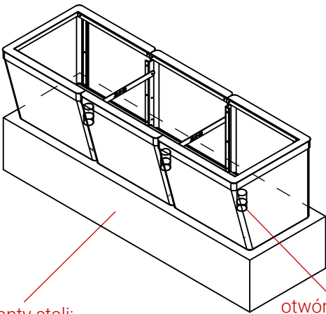
RZUT IZOMETRYCZNY
