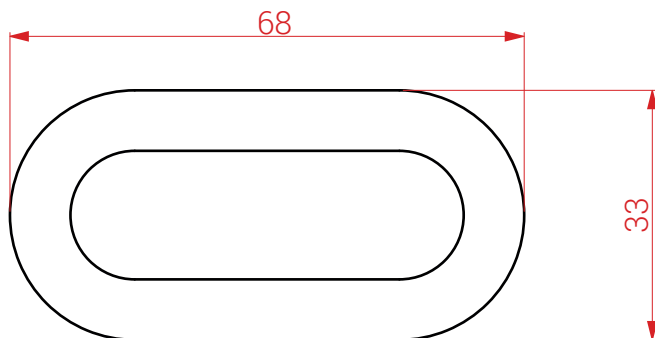
WIDOK Z TYŁU
