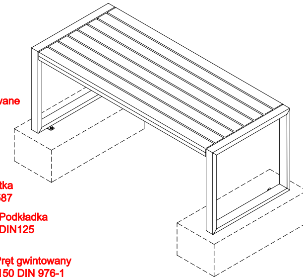
RZUT IZOMETRYCZNY
