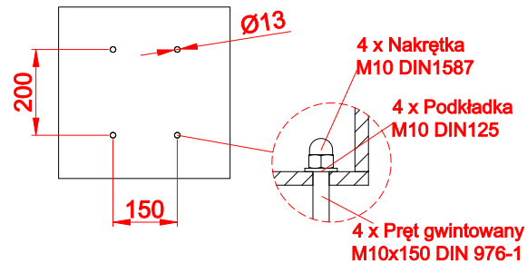
ROZSTAW OTWORÓW MONTAŻOWYCH
