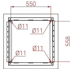
ROZSTAW OTWORÓW MONTAŻOWYCH
