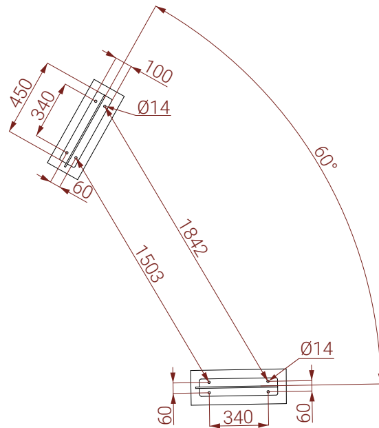
ESPACEMENT DES TROUS DE MONTAGE
