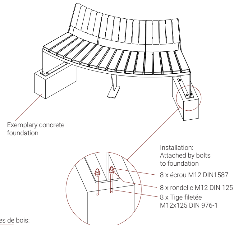
PROJECTION ISOMÉTRIQUE
