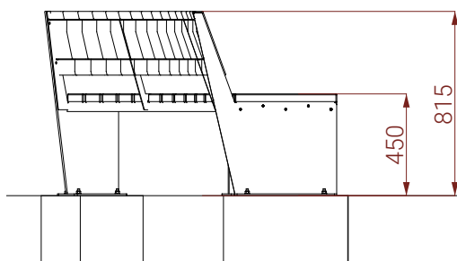
VUE LATÉRALE
