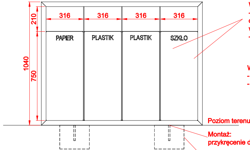
WIDOK Z FRONTU
