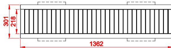
WIDOK Z GÓRY
