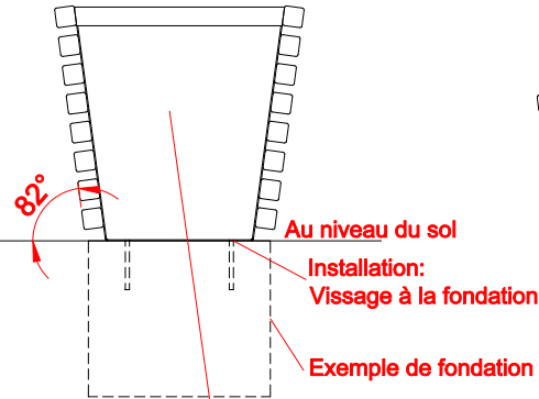
VUE LATÉRALE
