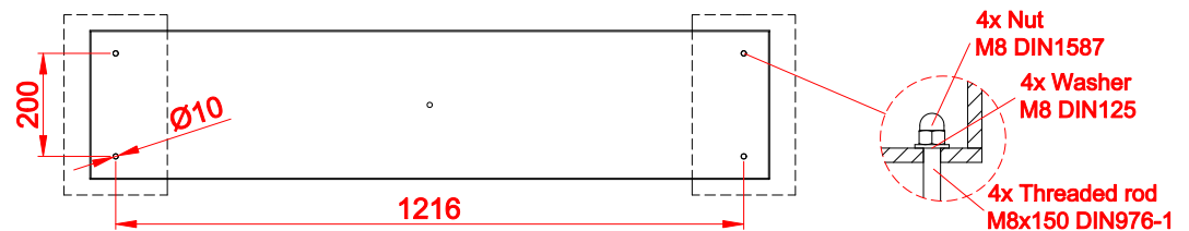
ESPACEMENT DES TROUS DE MONTAGE
