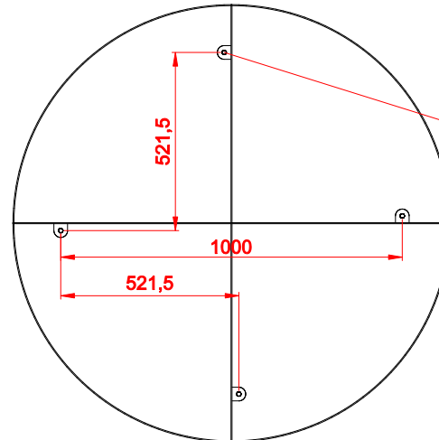
ROZSTAW OTWORÓW MONTAŻOWYCH
