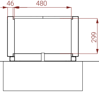
COUPE VERTICALE
