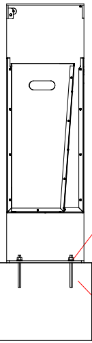
PRZEKRÓJ
