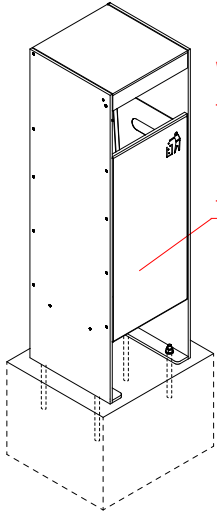
RZUT IZOMETRYCZNY
