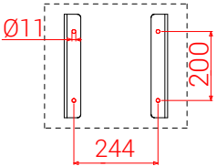
ROZSTAW ŚRUB MONTAŻOWYCH
