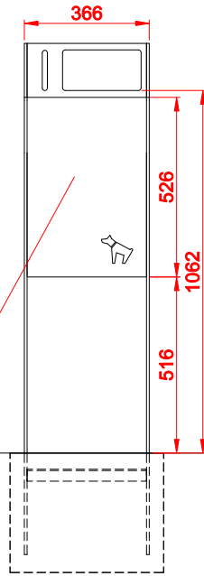
WIDOK Z FRONTU
