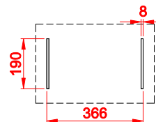
ROZSTAW OTWORÓW MONTAŻOWYCH
