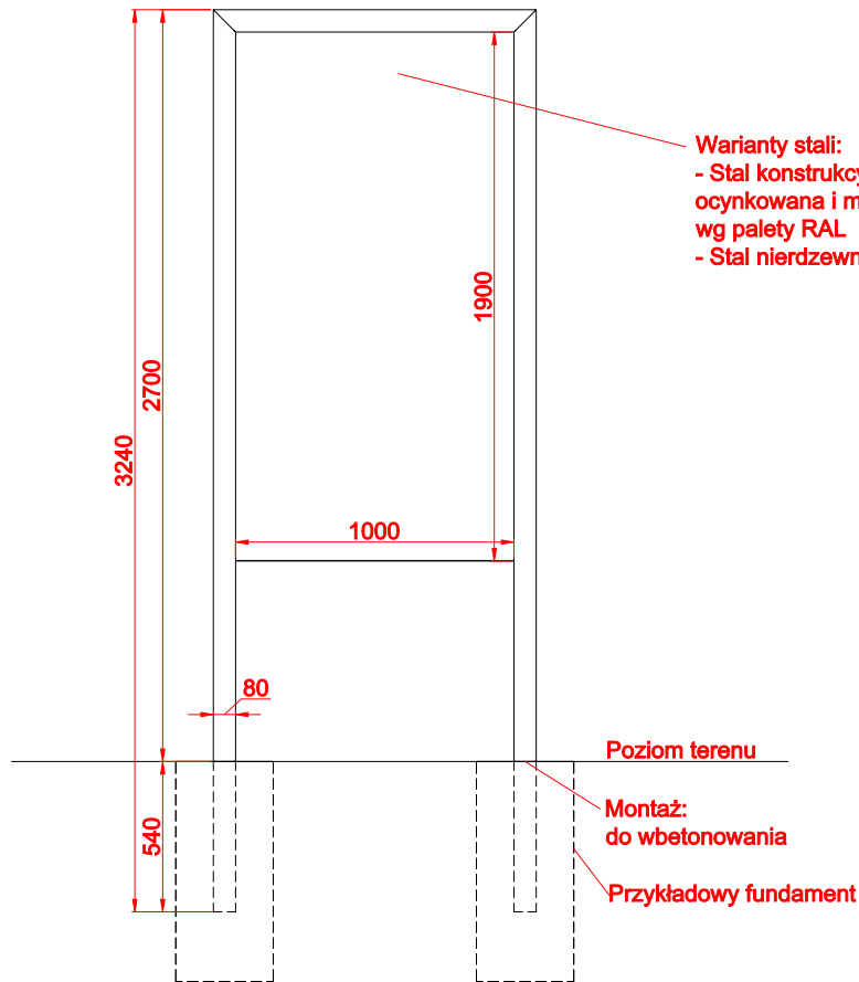
WIDOK Z FRONTU
