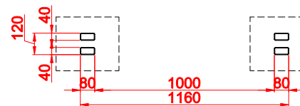
ROZSTAW OTWORÓW MONTAŻOWYCH
