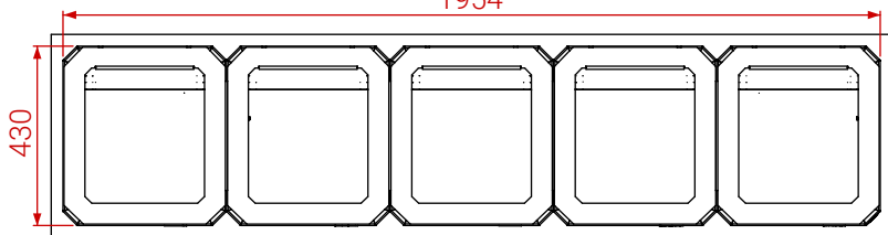
ROZSTAW OTWORÓW MONTAŻOWYCH (WIDOK Z GÓRY)
