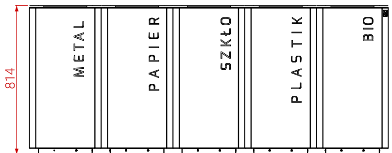
WIDOK Z FRONTU
