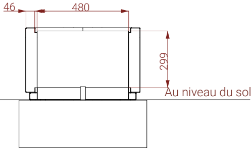
COUPE VERTICALE
