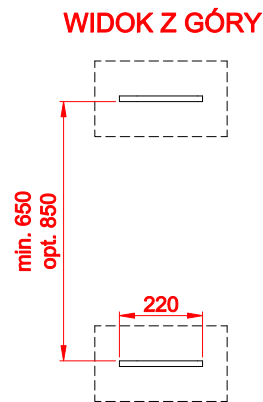
ROZSTAW OTWORÓW MONTAŻOWYCH
