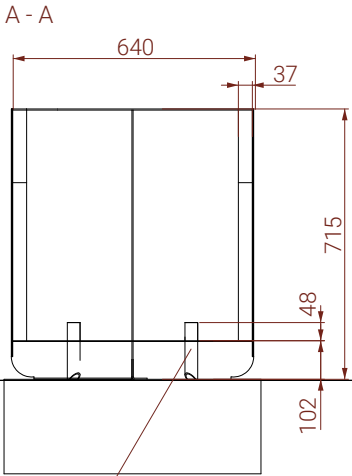
PRZEKRÓJ
