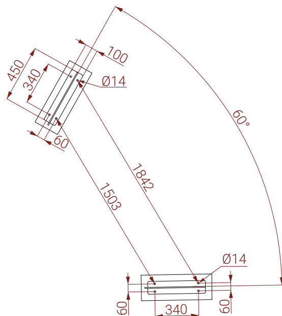
ROZSTAW OTWORÓW MONTAŻOWYCH
