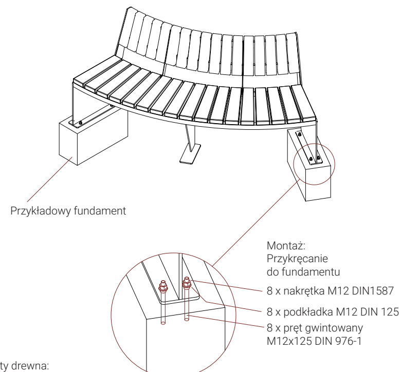
RZUT IZOMETRYCZNY
