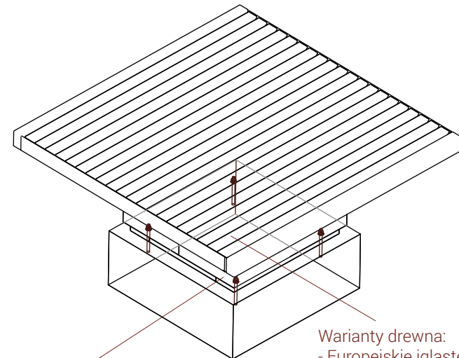
RZUT IZOMETRYCZNY
