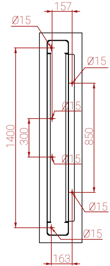
ESPACEMENT DES TROUS DE MONTAGE (FRAIS GÉNÉRAUX)
