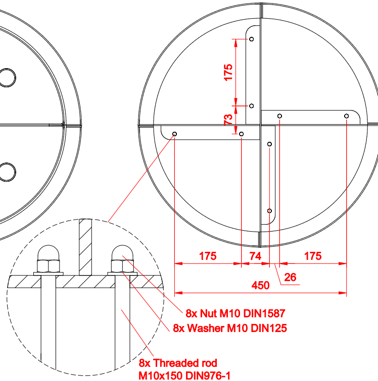
ESPACEMENT DES TROUS DE MONTAGE
