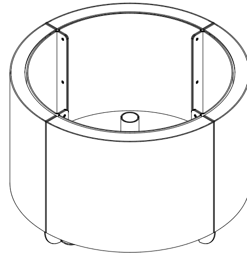
PROJECTION ISOMÉTRIQUE
