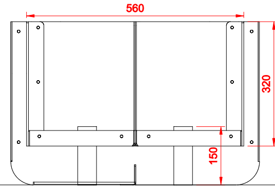
COUPE VERTICALE
