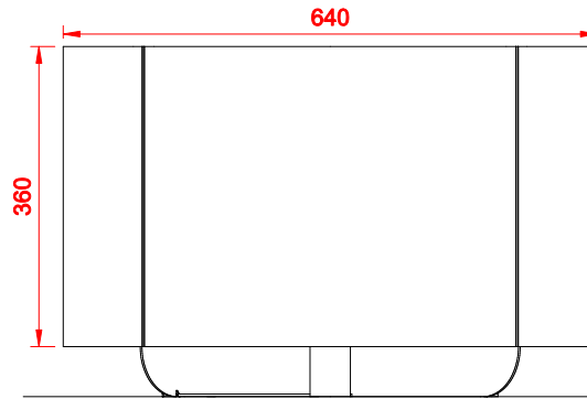
VUE LATÉRALE
