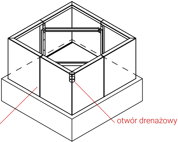
RZUT IZOMETRYCZNY
