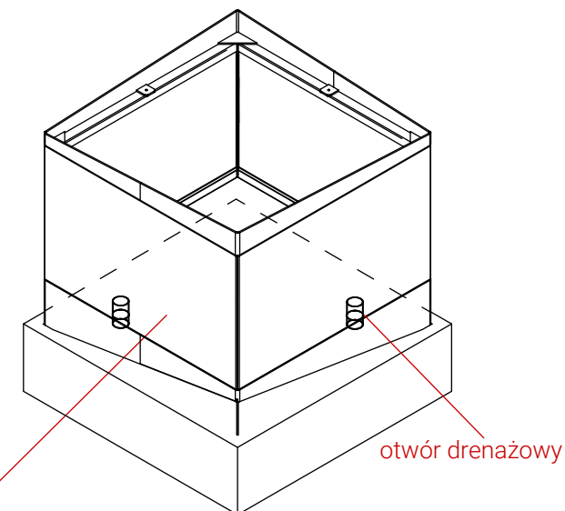
RZUT IZOMETRYCZNY
